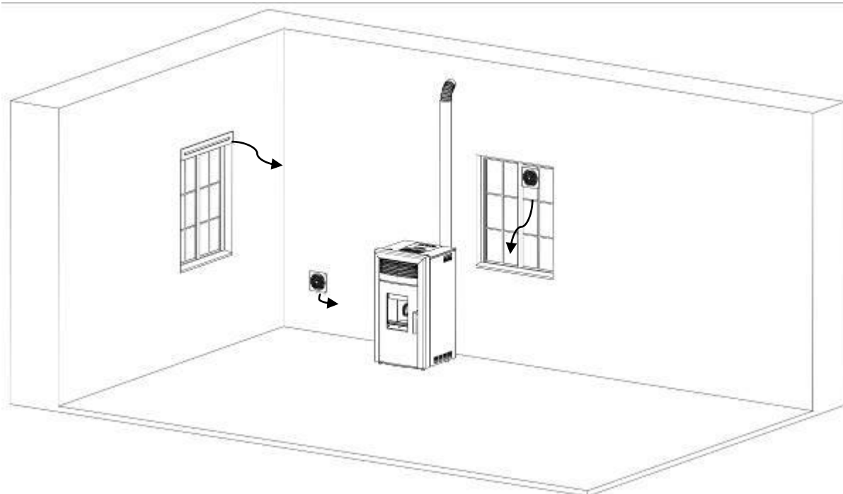
Přívod čerstvého vzduchu do místnosti, kde jsou kamna instalována
