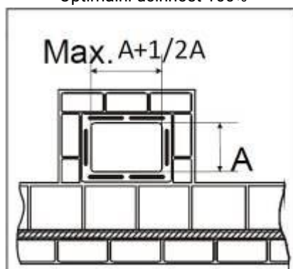
Je zakázáno používat komínové trubky s vnitřní pravoúhlou částí, které se liší od plánu. Účinnost pouhých 40%%
